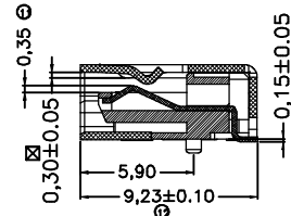
SEC. A-A
